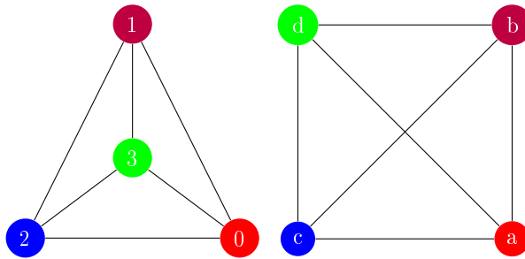
Figura 1.5: Grafs isomorfs
