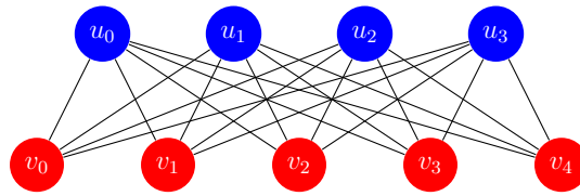
Figura 1.10: Graf bipartit complet K_{4,5}
