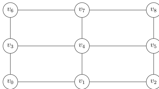
Figura 1.12: Graf xarxa G_{3,3}
