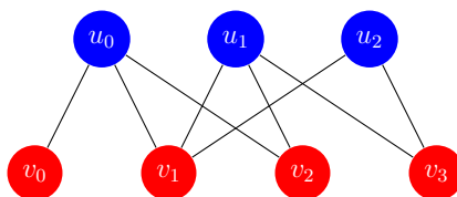
Figura 1.9: Graf bipartit
