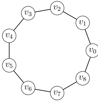
Figura 1.7: Cicle C_9
